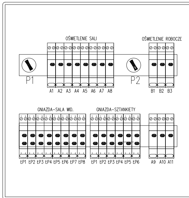
(ROZDZIELNICA RN-2x18-55 FIRMY LEGRAND-FAEL wys.=416/szer.=402/gł.148)
